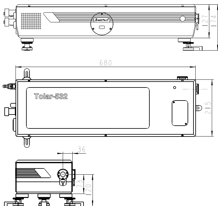
Tolar-532-50激光头
